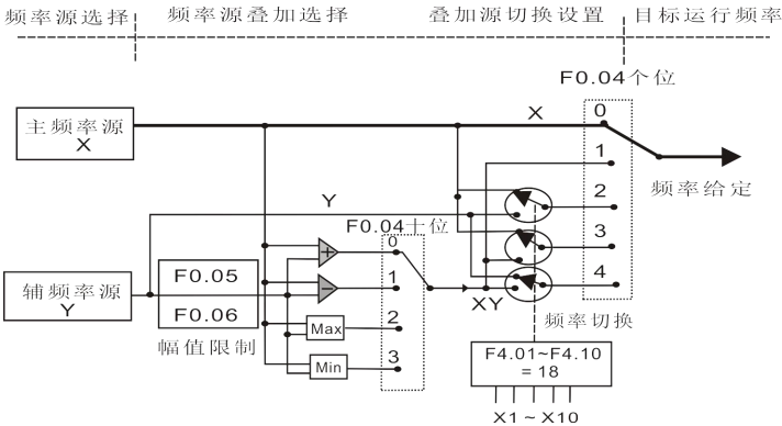
图 6-1 频率叠加图
