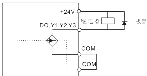
图3-16 数字输出端子接线示意图
