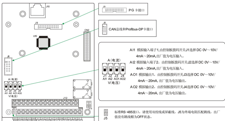
图3-9 控制回路端子布置图
