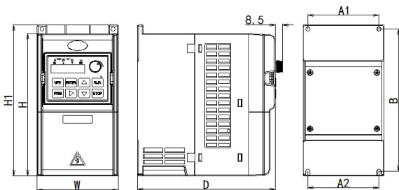
图2-4 22kW及以下功率段外形尺寸及安装示意图
