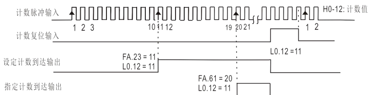
图6-25 设定计数值给定和指定计数值给定示意图
