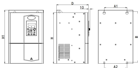
图2-5 30kW~110kW外形尺寸及安装尺寸示意图
